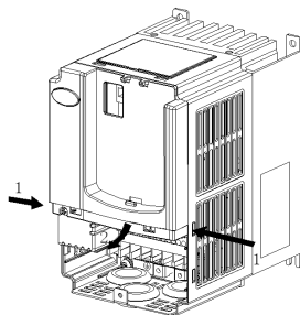
图 2-6 上盖板的拆卸
