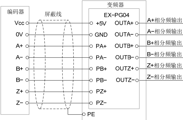
EX-PG04 卡采用内部电源的连接示意图
