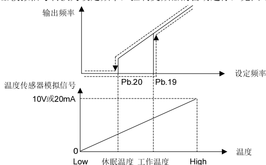
图 6-37 零频运行上下界
