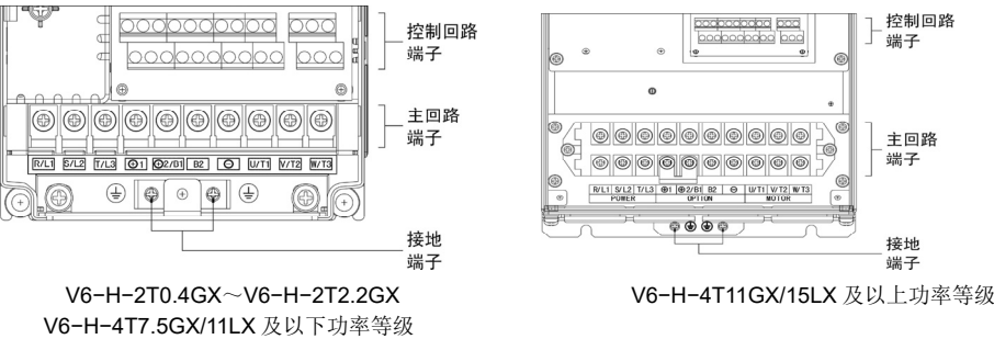
图 3-2 产品端子配置情况
