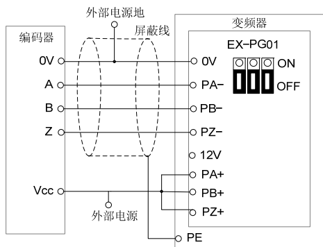
EX-PG01 卡采用外部电源的连接示意图（跳线跳到 OFF 侧）
