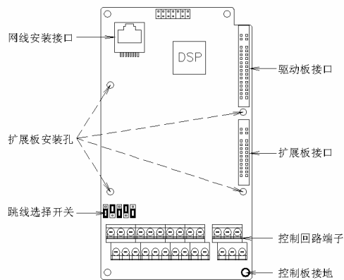
图 3-7 控制板示意图
