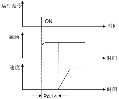
图 6-39 预激磁
