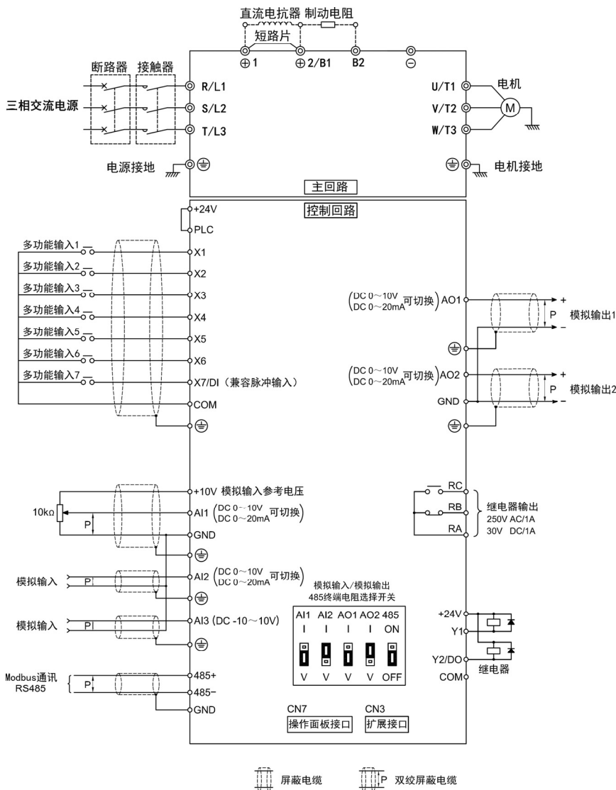
图 3-6 端子配线图 (以 V6-H-4T5.5GX/7.5LX 型举例)
