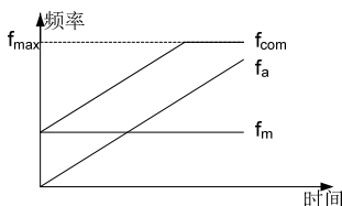
图 6-4 开环主辅给定运算 0
