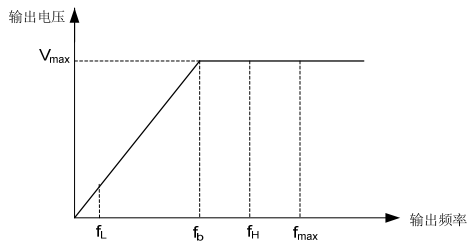
图 6-2 特性参数定义
