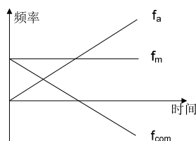
图 6-5 开环主辅给定运算 1
