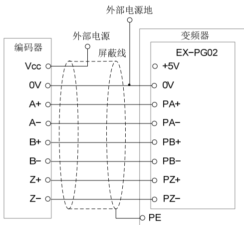
EX-PG02 卡采用外部电源的连接示意图
