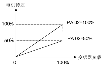
图 6-34 矢量控制 1 转差补偿增益
