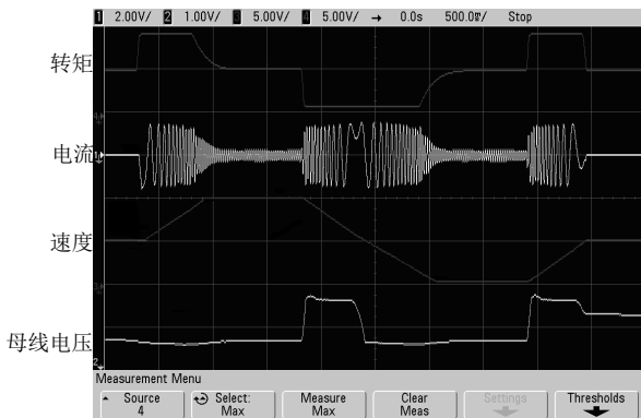
图 1 0Hz→正转 50Hz→0Hz→反转 50Hz→0Hz 的急加减速四象限运行
