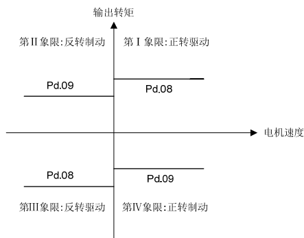
图 6-38 转矩限定
