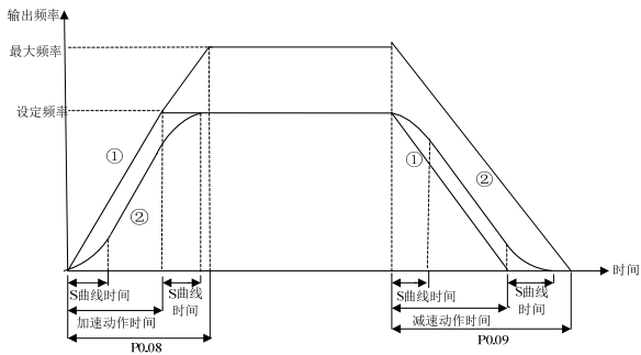
图 6-1 加减速时间及 S 段曲线
