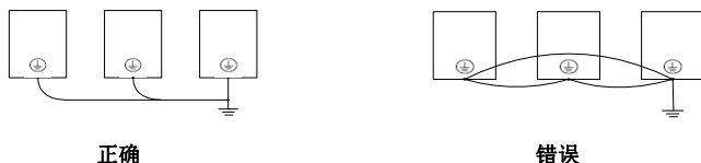
图 3-3 接地线配线
