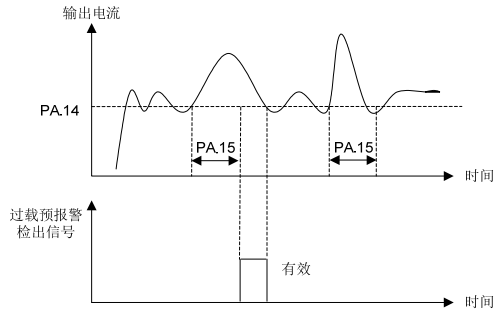
图 6-35 过载预警检出信号
