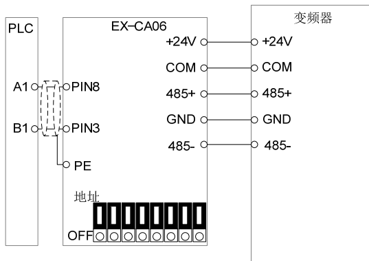
EX-CA06 卡连接示意图
