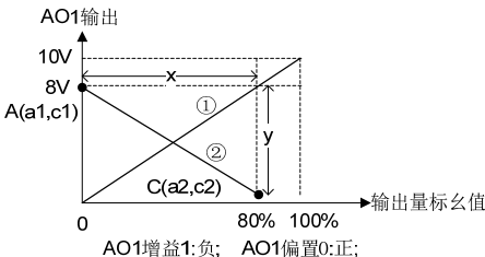
图 6-29 AO1 特性曲线 kx+b
