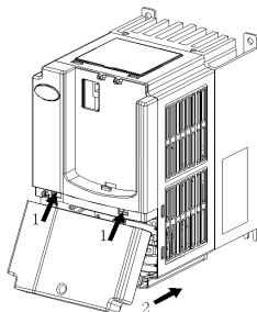
图 2-8 下盖板的安装
