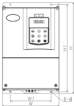
V6-H-4T11GX/15LX 及以上功率等级
