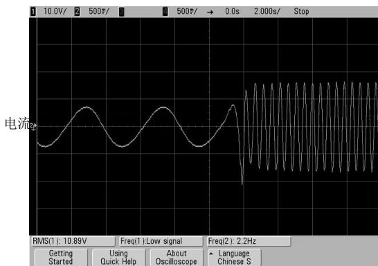
图 3 无速度传感器矢量控制下 0.25Hz 突加满载运行
