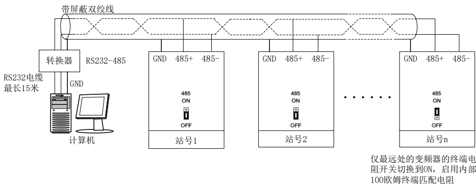
附图 4 多台变频器与计算机的连接
