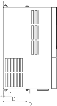
V6-H-4T11GX/15LX 及以上功率等级
