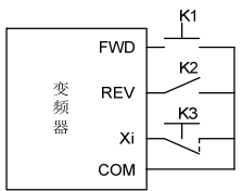
图 6-17 三线式运行模式 2
