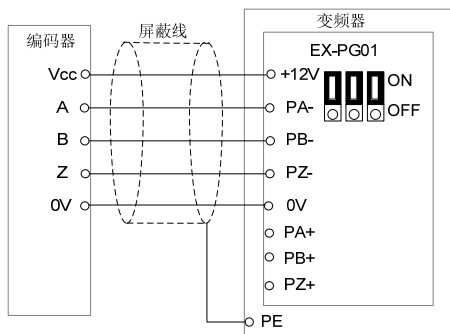
EX-PG01 卡采用内部电源的连接示意图（跳线跳到 ON 侧）
