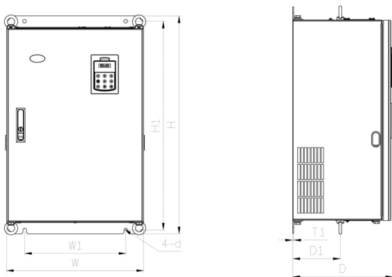
V6-H1-4T132G 及以上功率等级
