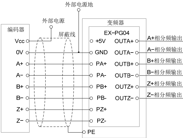
EX-PG04 卡采用外部电源的连接示意图
