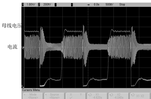
图 2 任意加减速和稳态运行，电流电压控制稳定不会跳闸保护
