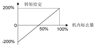
图 6-25 转矩给定 2
