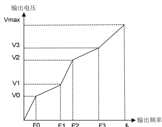
图 6-13 多段 V/F 曲线
