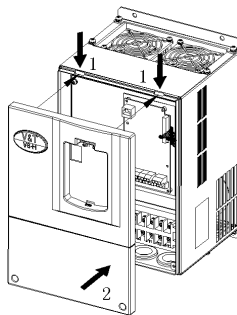
图 2-10 安装盖板
