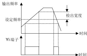
图 6-30 频率到达信号 FAR
