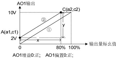
图 6-26 AO1 特性曲线 kx+b
