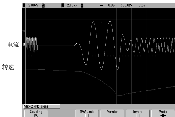
图 5 电机高速自由旋转时跟踪并降频后平滑起动
