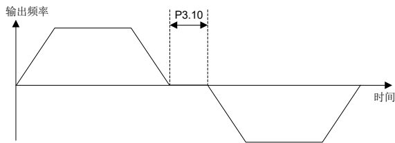
图 6-11 正反转死区时间
