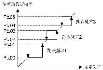
图 6-36 跳跃频率上下限
