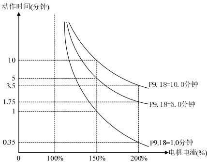
图 6-33 电机过载保护特性曲线（恒转矩）
