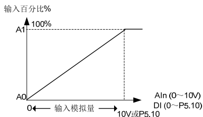
图 6-19 输入模拟量（电压/频率）对应百分比
