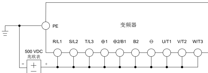
图8-1 V6-H-2T0.4GX~V6-H-2T2.2GX 、V6-H-4T0.75GX/1.5LX~V6-H-4T15GX/18.5LX 主回路绝缘测试
