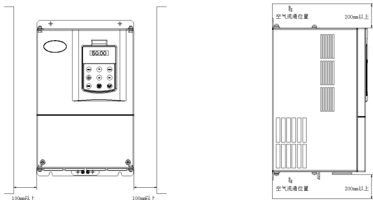
图 2-2 V6-H-4T11GX/15LX 及以上功率等级的安装方向和空间
