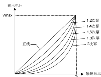
图 6-12 V/F 曲线
