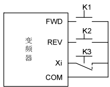
图 6-16 三线式运行模式 1
