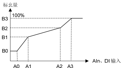
图 6-23 输入模拟量特性曲线
