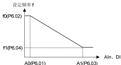
图 6-22 设定频率特性曲线（反作用）
