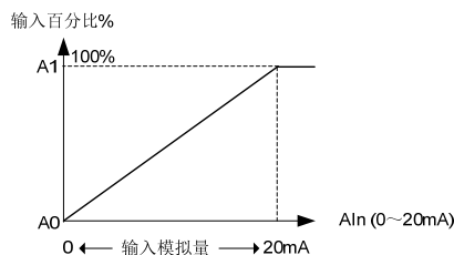
图 6-20 输入模拟量（电流）对应百分比
