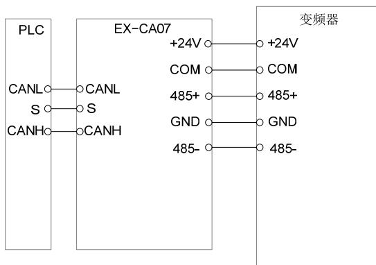
EX-CA07 卡连接示意图
