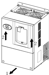
图 2-9 拆卸盖板
