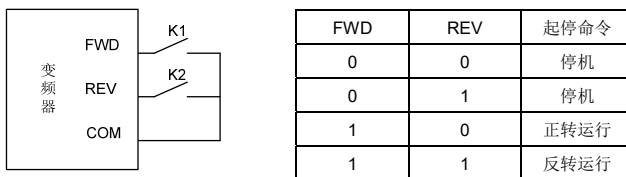
图 6-15 两线式运行模式 2
