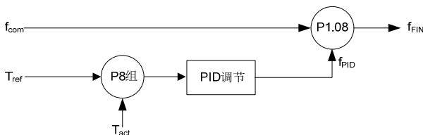
图 6-10 开环和闭环复合运行给定
