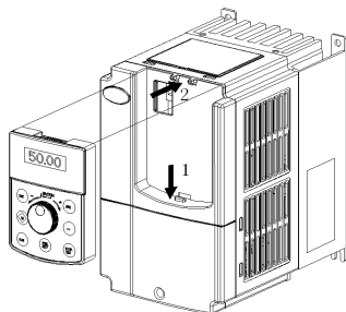
图 2-4 操作面板的安装
