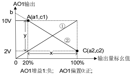
图 6-28 AO1 特性曲线 kx+b
