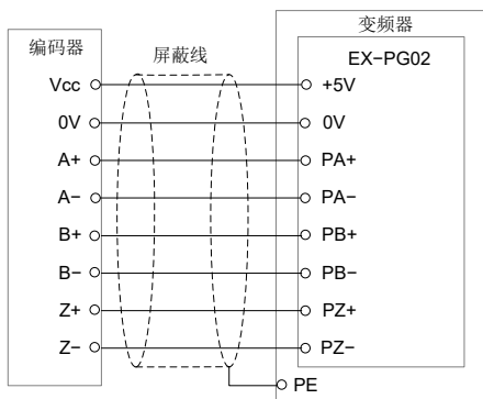
EX-PG02 卡采用内部电源的连接示意图
