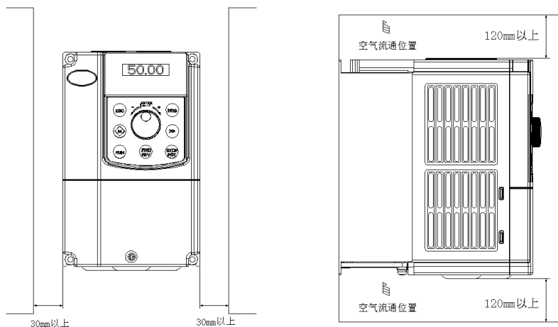
图 2-1 V6-H-2T0.4GX~V6-H-2T2.2GX 和 V6-H-4T7.5GX/11LX 及以下功率等级的安装方向和空间
