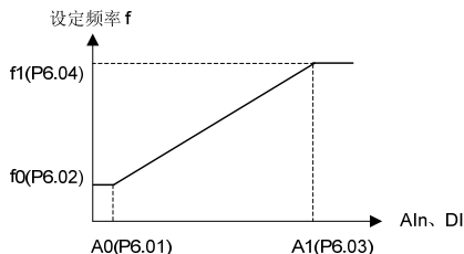
图 6-21 设定频率特性曲线（正作用）
