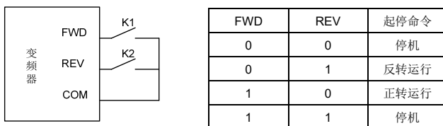
图 6-14 两线式运行模式 1
