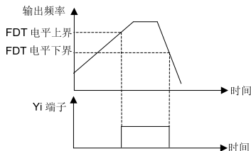
图 6-31 频率水平检测信号 FDT
