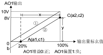
图 6-27 AO1 特性曲线 kx+b
