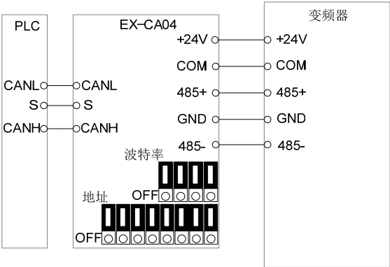
EX-CA04 卡连接示意图
