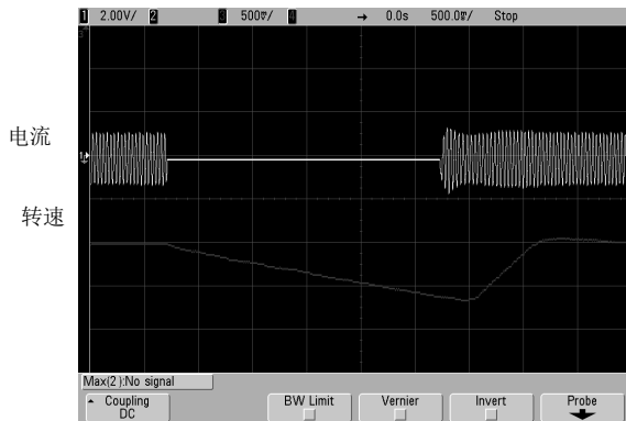
图 4 电机自由旋转时快速无冲击的转速跟踪
