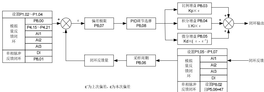
图 6-32 PID 原理框图
